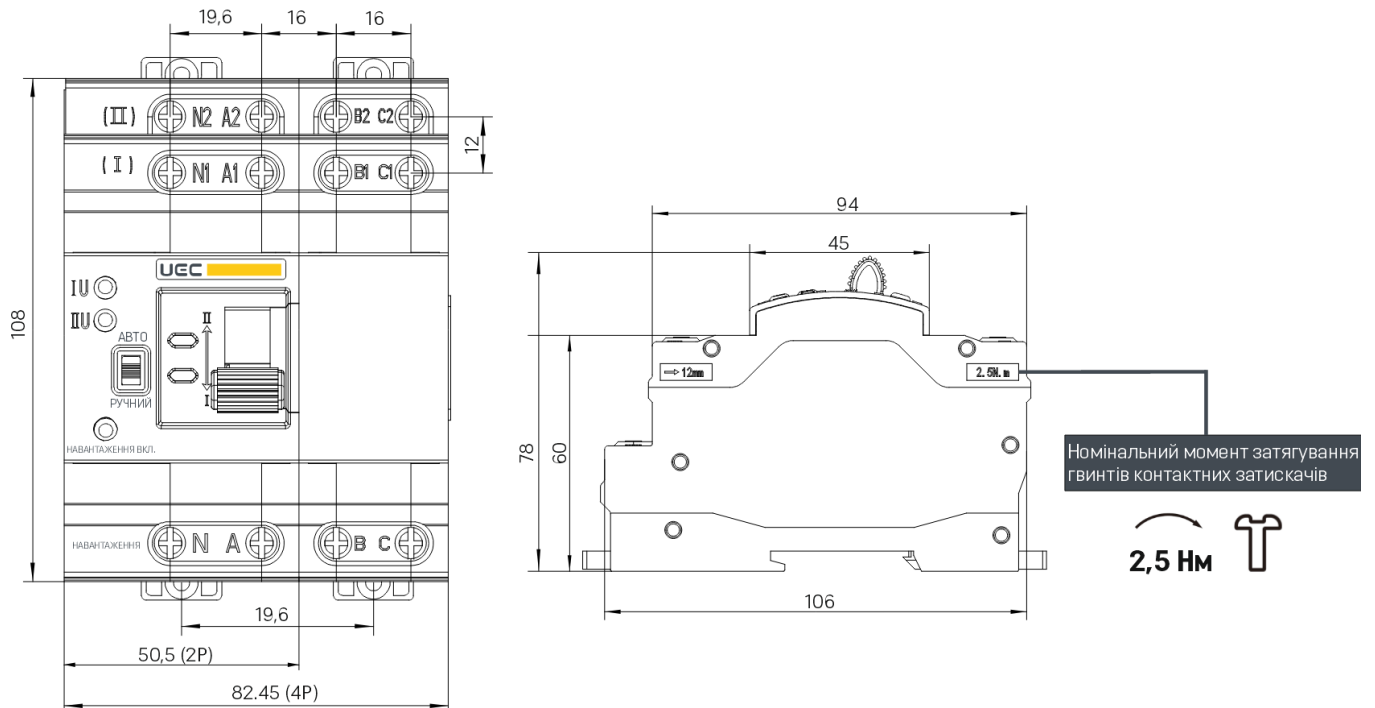
Рисунок 1 – Габаритні розміри перемикачів
