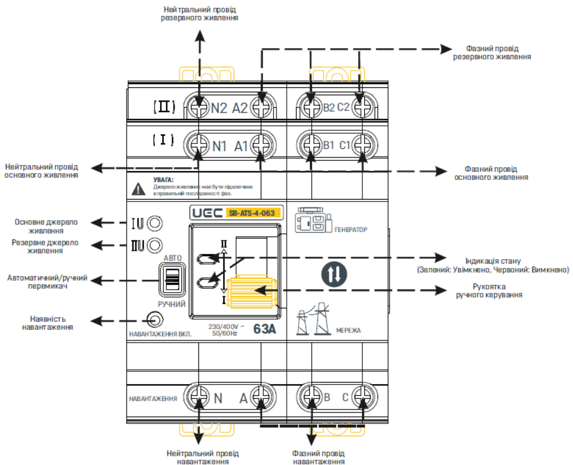
Рисунок 2 – Підключення перемикача
