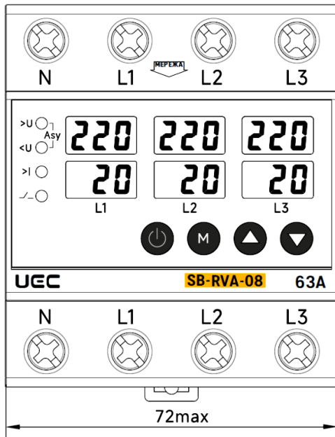
Рисунок 4 – Габаритні та установчі розміри реле контролю напруги та струму SB-RVA-08-4.
