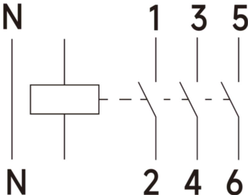
Рисунок 5 — Схема електрична реле контролю напруги та струму SB-RV-08-4.
