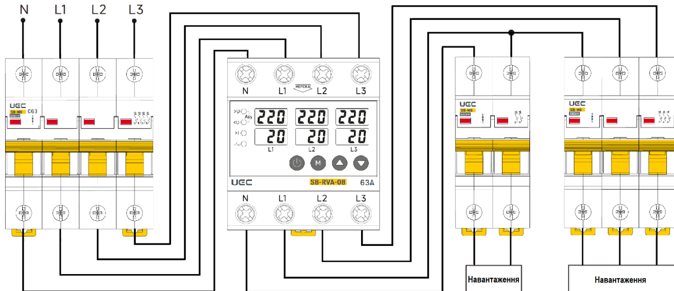
Рисунок 6 - Рекомендована схема підключення реле напруги та струму SB-RVA-08-4.
