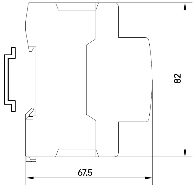
Рисунок 4 – Габаритні та установчі розміри реле контролю напруги та струму SB-RVA-08-4.
