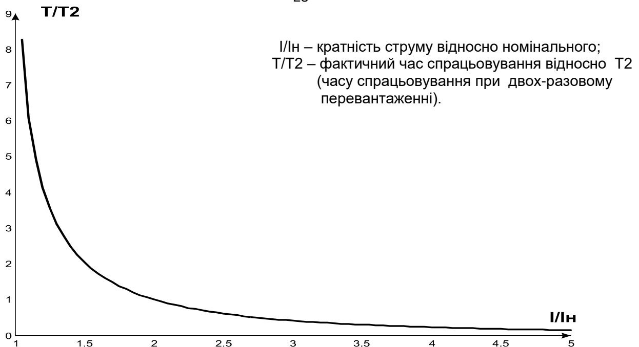
Рисунок 3.4 - Струмо-часова характеристика
