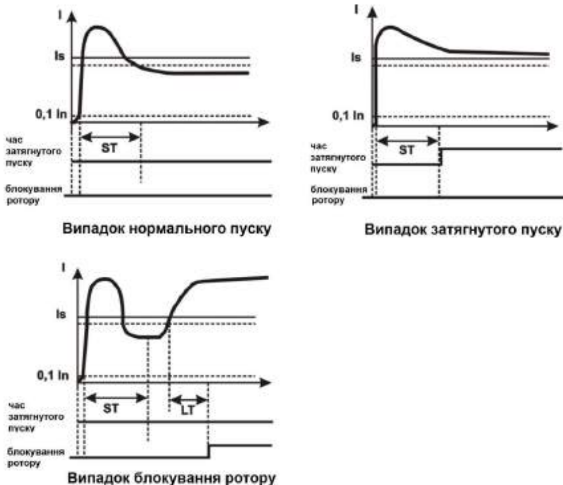
Рисунок 3.3 - Затягнутий пуск та блокування ротора
