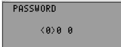
Рисунок 5.8 - Пароль налагоджувальника
