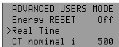
Рисунок 5.9 - Рівень налагоджувальника
