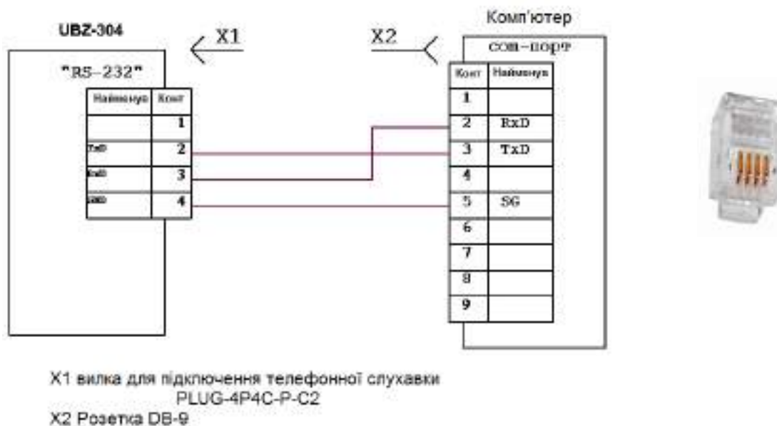
Рисунок 5.12 - Схема підключення UBZ-304 до ПК
