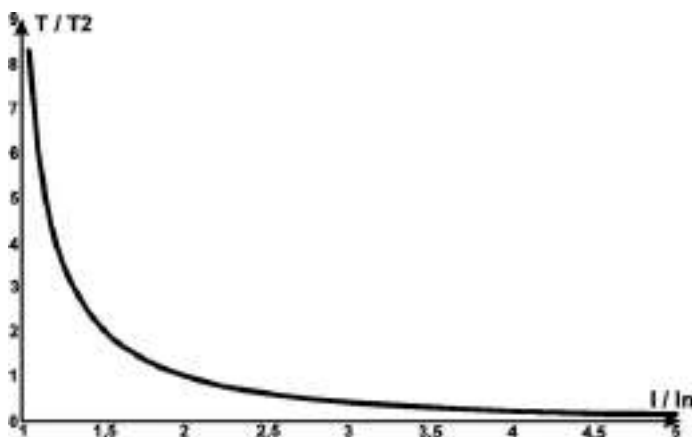
Рисунок 7 – Токо-временная характеристика
