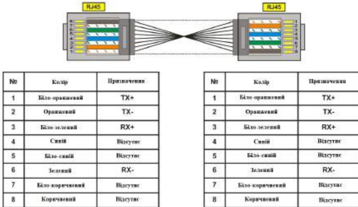
Рисунок 5.3 – Нумерація виводів кабелю з'єднання з мережею Ethernet
