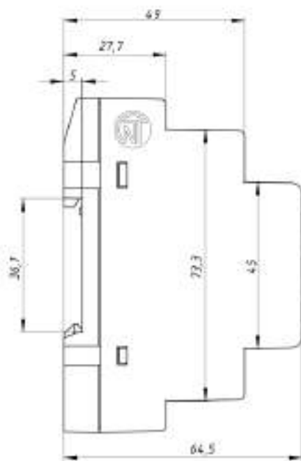
Рисунок 1 – Органи керування, габаритні та установчі розміри RNPP-311M
