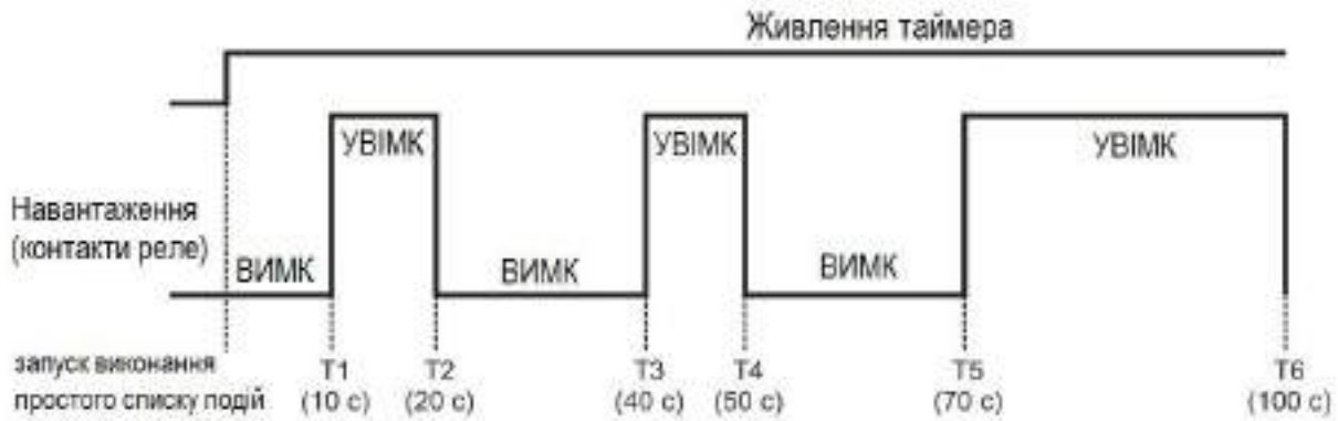
Рисунок 3.6 – Увімкнення навантаження на прикладі простого режиму роботи
