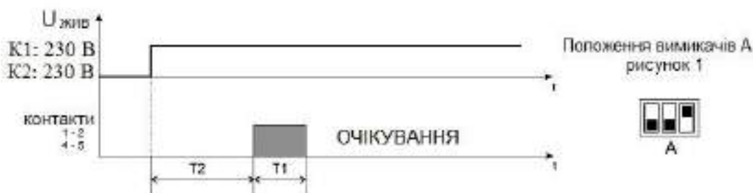
Рисунок 3 – Алгоритм роботи реле «Імпульсний 1»
