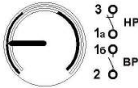
Рисунок 3 – Схема підключення датчика тиску
