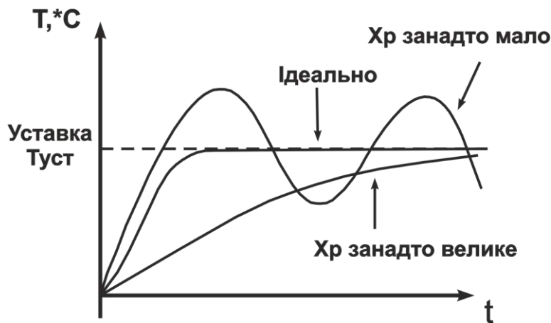
Рисунок 3.8 - Графік роботи пропорційного регулятора
