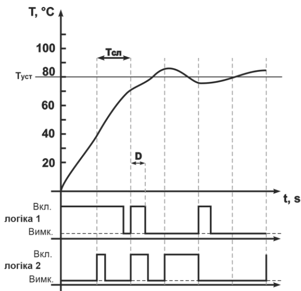
Рисунок 3.11 - Діаграма спрацьовування вихідних реле в режимі ПІД-регулювання
