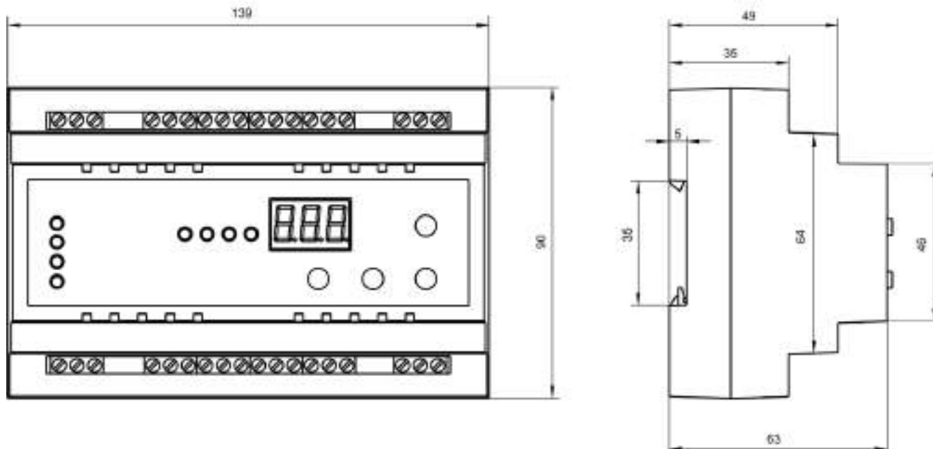
Рисунок 3.1 - Габаритні розміри приладу
