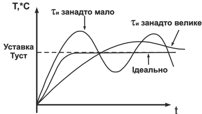
Рисунок 3.9 – Графік роботи інтегрального регулятора
