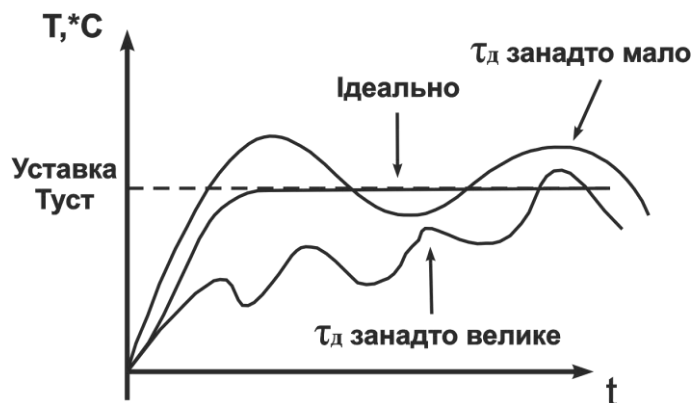
Рисунок 3.10 – Графік роботи диференціального регулятора
