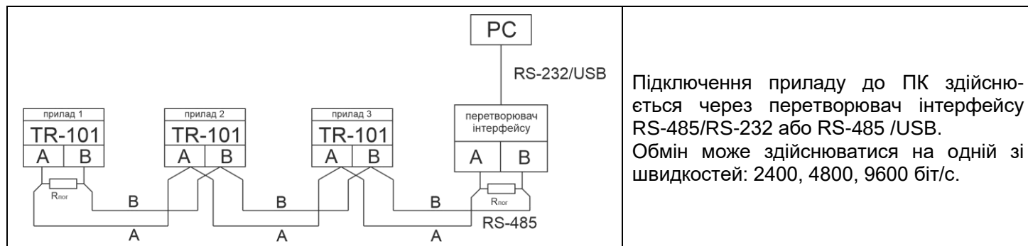
Рисунок А1 - Підключення приладів у мережу RS-485
