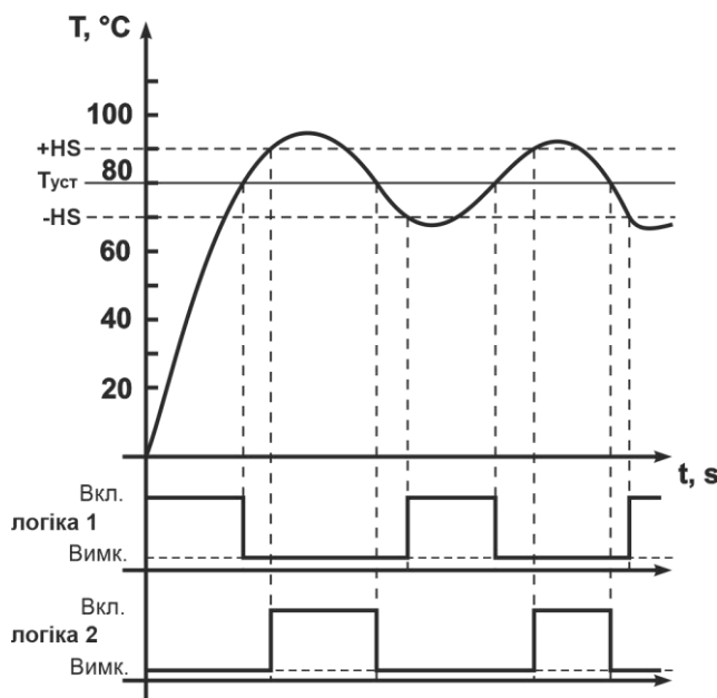
Рисунок 3.7 – Діаграма спрацьовування вихідних реле в режимі двопозиційного регулювання
