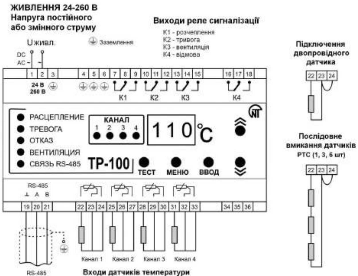
Рисунк 2 - Електричні з'єднання TP-100
