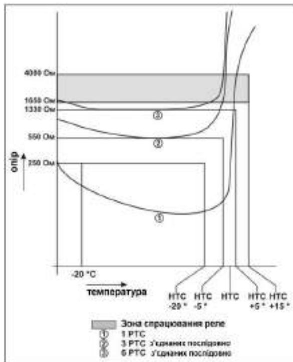
Рисунок 3 - Графік залежності опору від температури PTC датчиків
