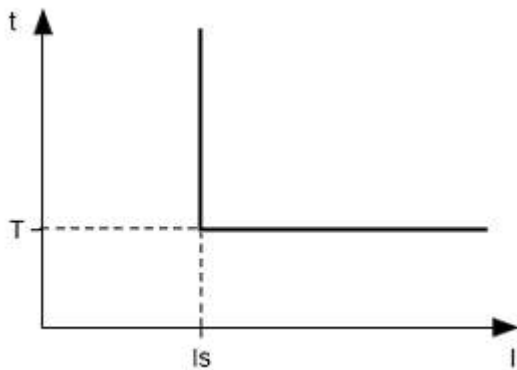
Рисунок 3.1 – Принцип захисту з незалежною витримкою часу
