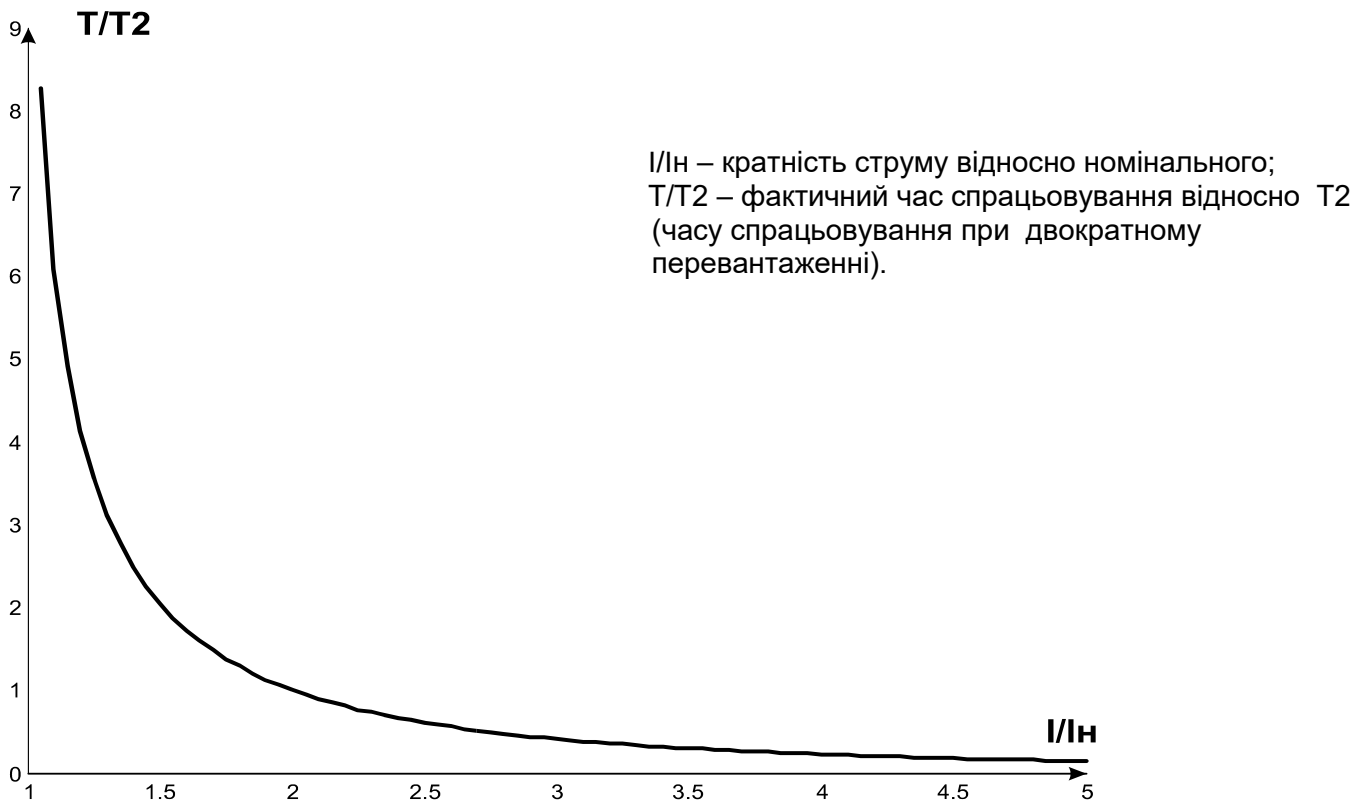
Рисунок 3.4 – Струмо-часова характеристика
