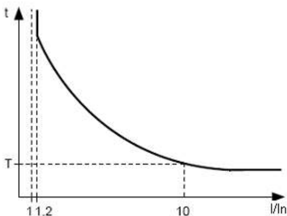
Рисунок 3.2 – Принцип захисту із залежною витримкою часу
