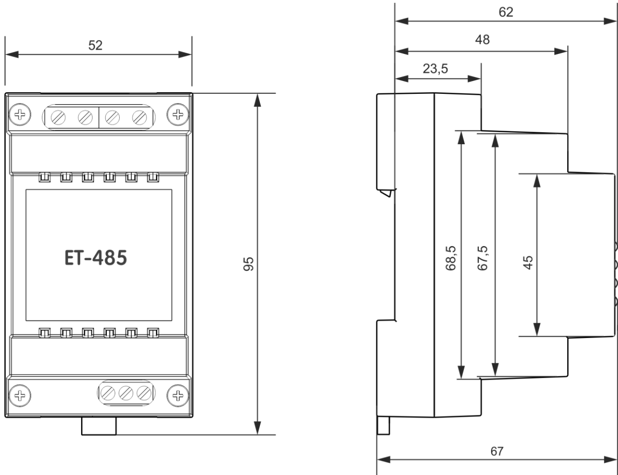
Рисунок 1 – Габаритні розміри виробу
