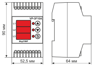
Габаритні розміри
