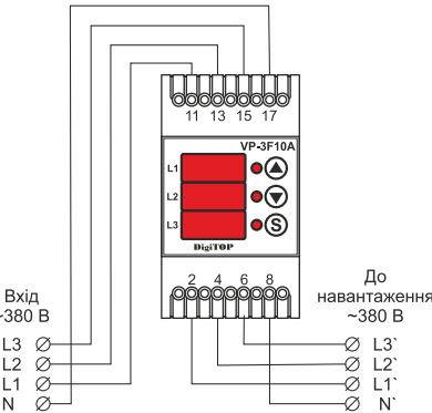
Схема підключення
