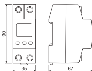
Габаритні розміри
