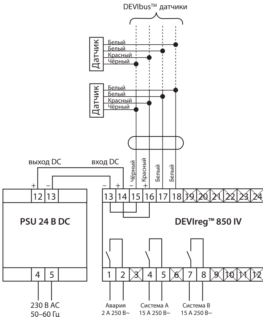
Рис. А - Схема соединений DEVlreg ™ 850
