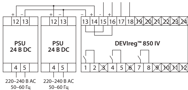
**Рис. Н — соединение 2 блоков PSU в параллель
